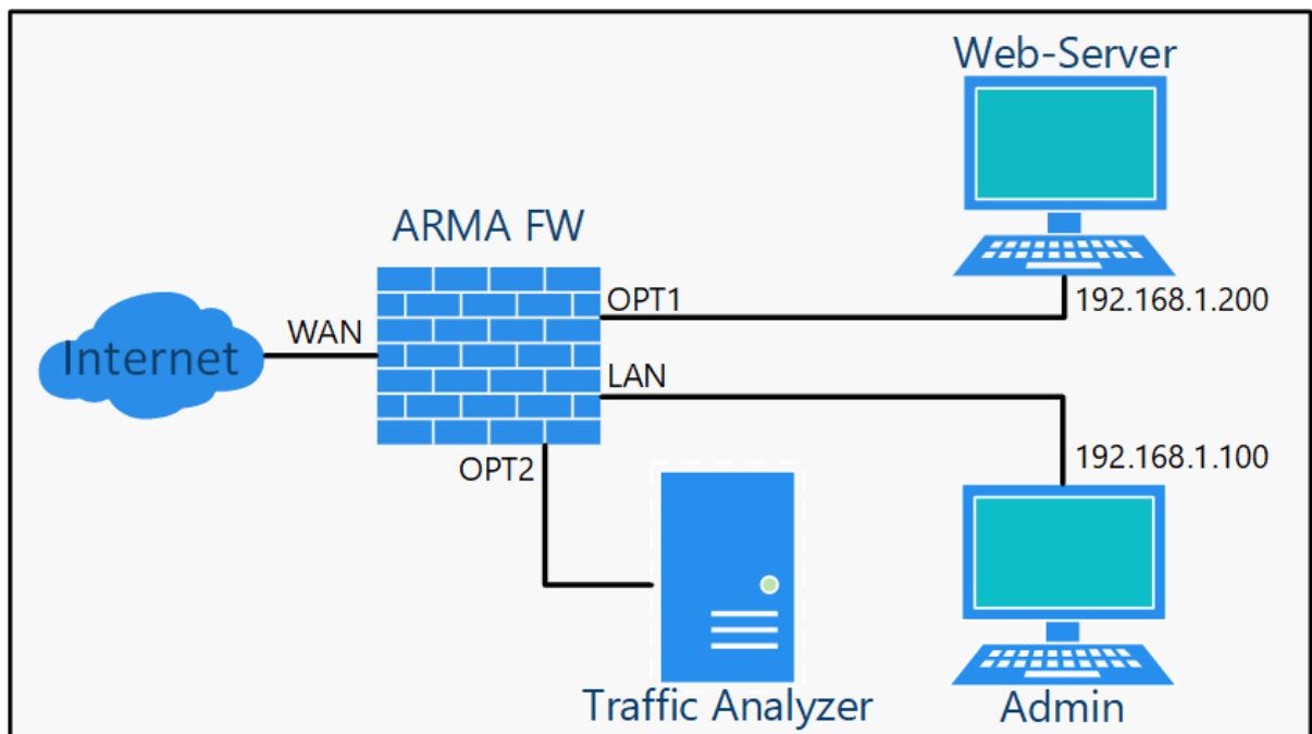
Рисунок – Стенд для настройки зеркалирования трафика
