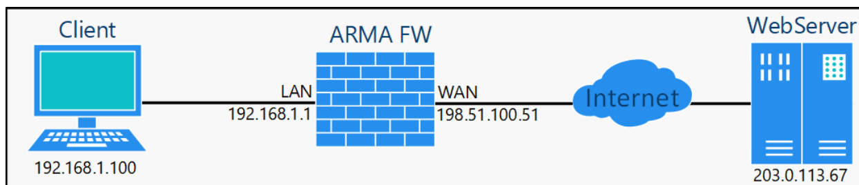
Рисунок – Схема стенда для настройки работы ARMA FW с родительским прокси-сервером
