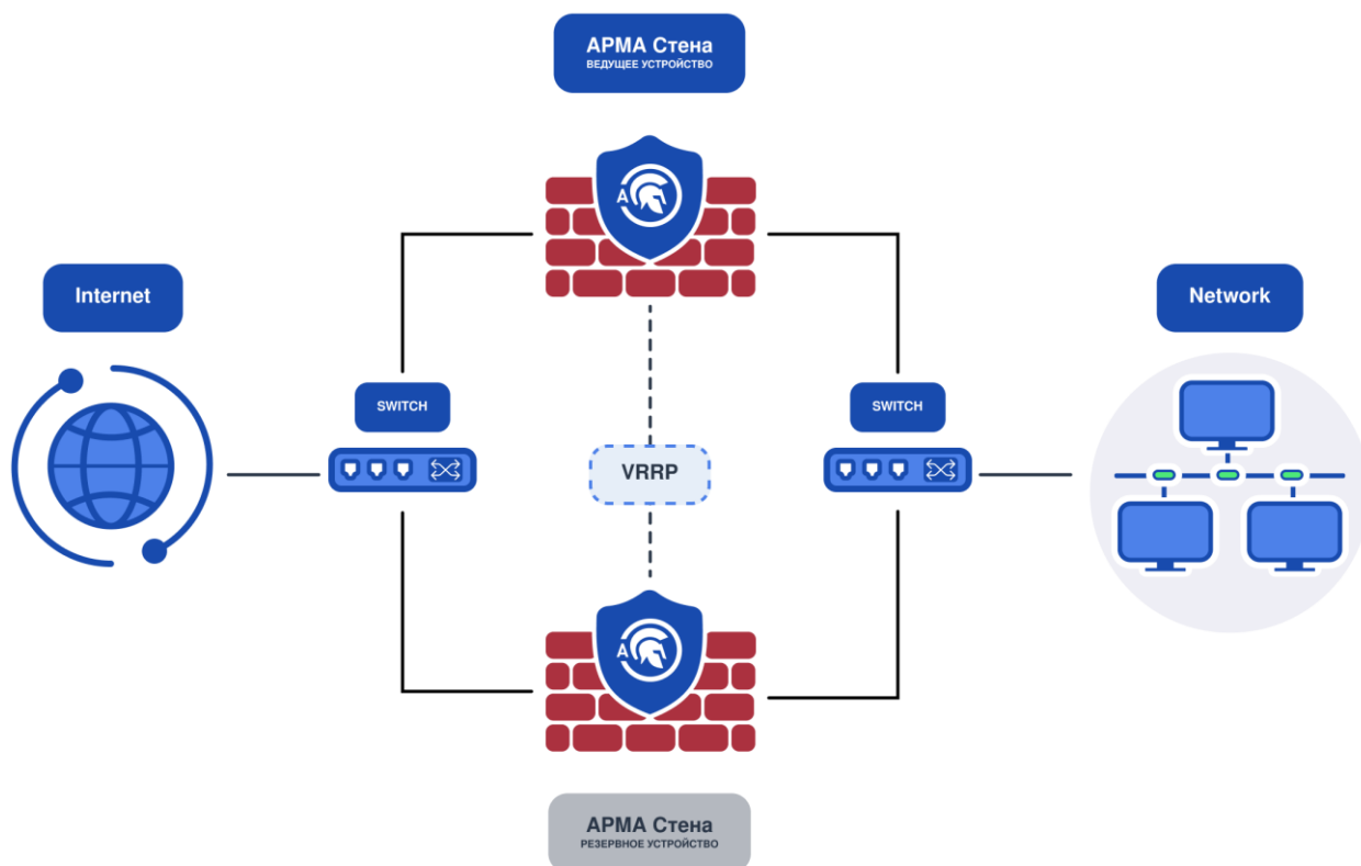
Рисунок – Режим отказоустойчивого кластера
