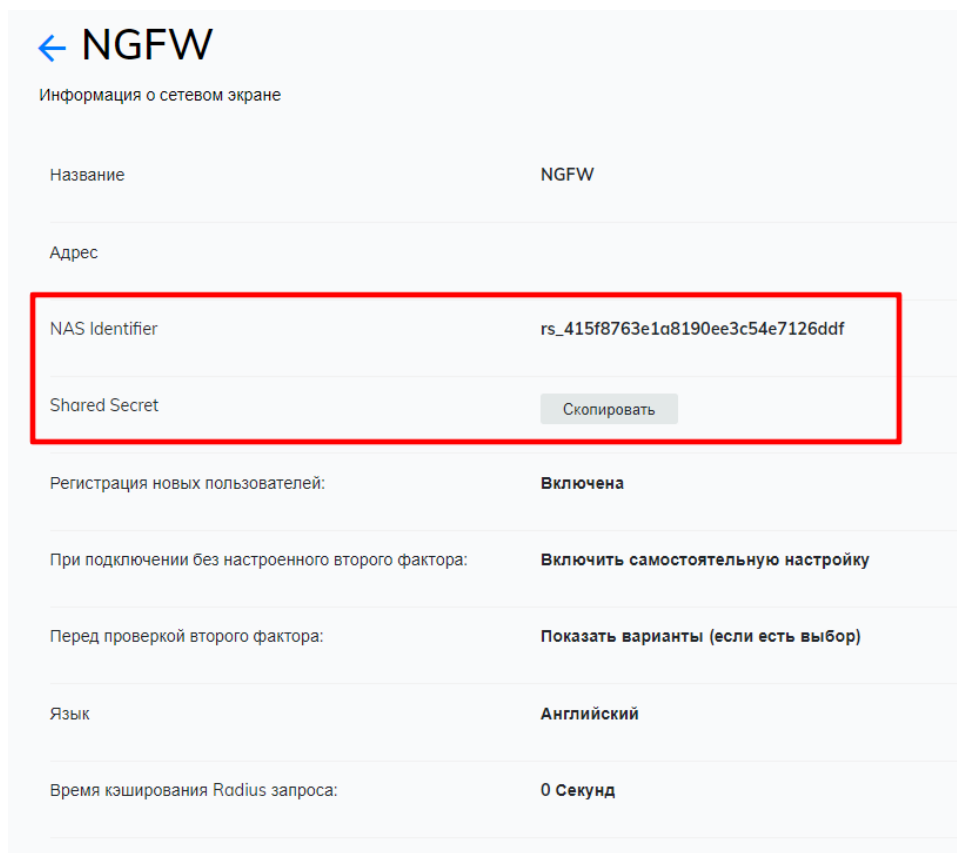
Рисунок – Параметры добавленного ресурса
