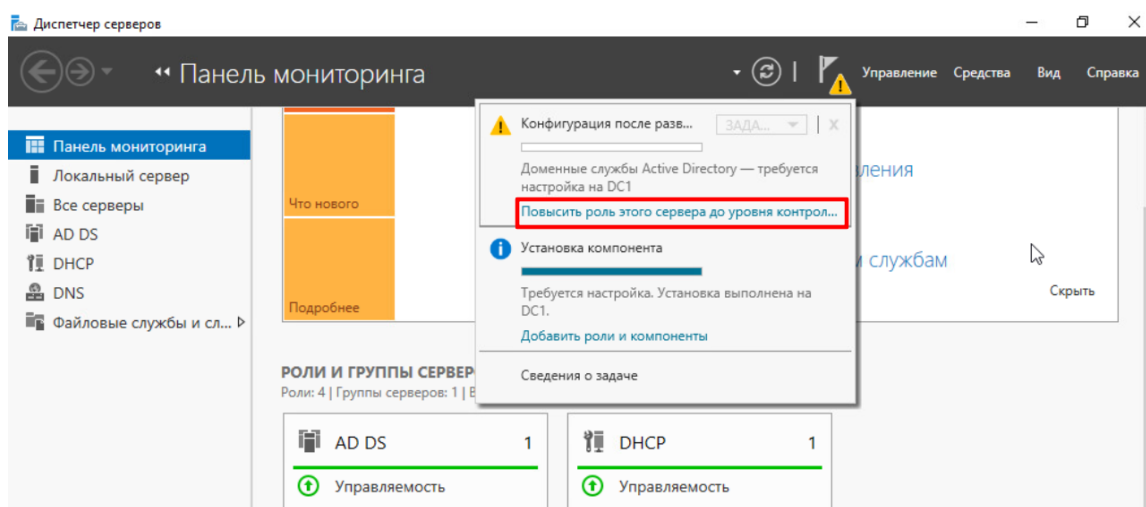
Рисунок – Настройка Active Directory
